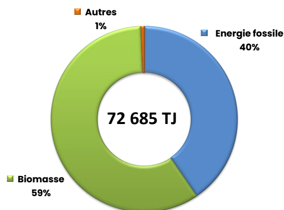
Consommation d'énergie primaire en 2022
